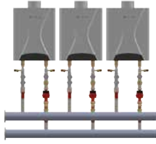
TKKS 003 KASKAD KAZAN ÜÇLÜ BAĞLANTI SETİ KASKAD BOILER TRIBLE CONNECTION
